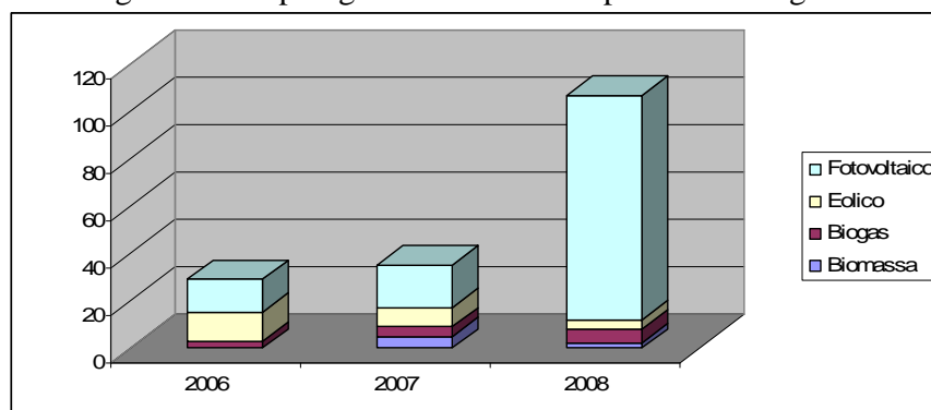
Fig. 6.1.9 – Tipologia di investimento per fonte energetica
